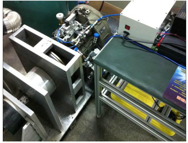
AMT 换挡气动伺服控制实验台架
