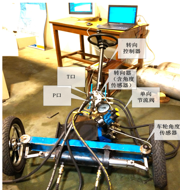
叉车电控全液压转向系统样机
