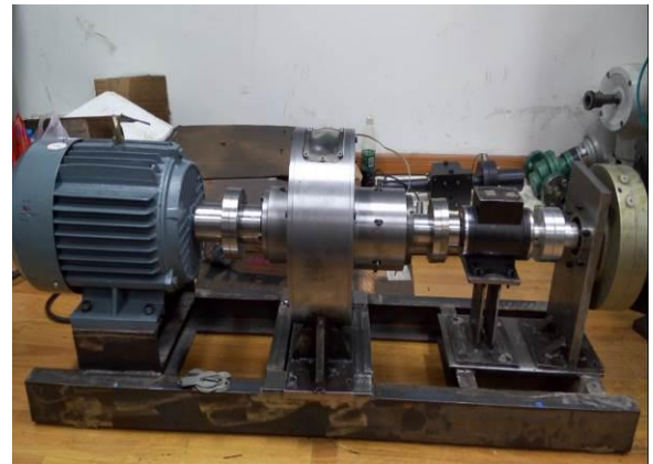
液粘/磁流变液调速离合器试验台
