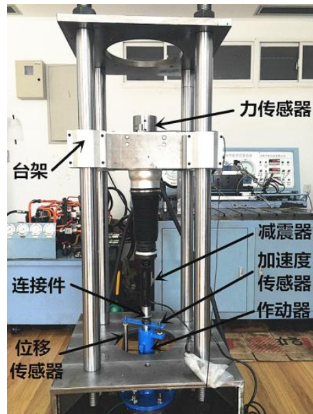
轿车用阻尼可调式液压减振器与试验装置
