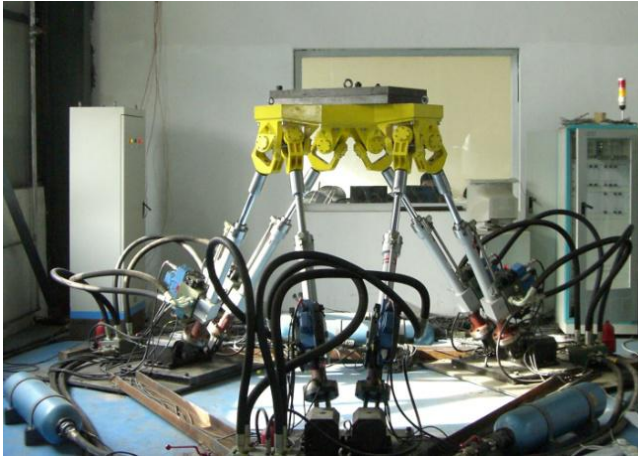
六自由度液压振动台
